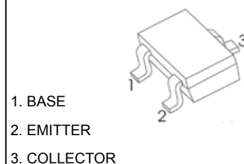
SOT-323
